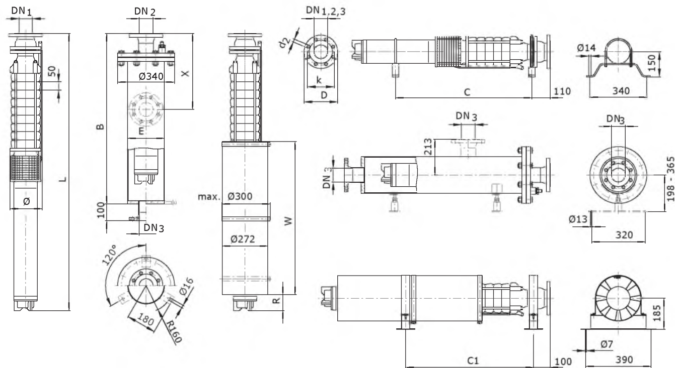
Чертеж с размерами Wilo-EMU KD 25
