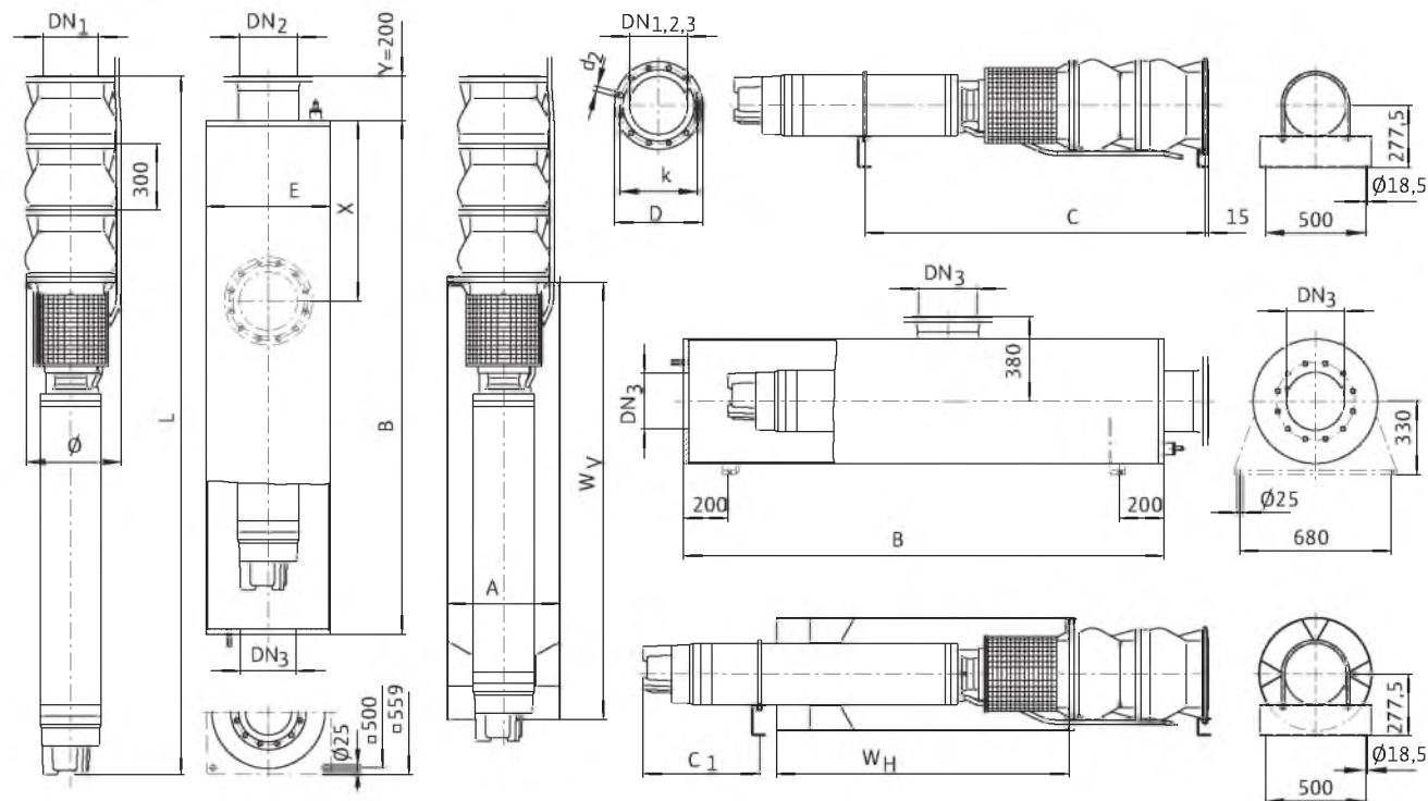
Чертеж с размерами Wilo-EMU D 500
