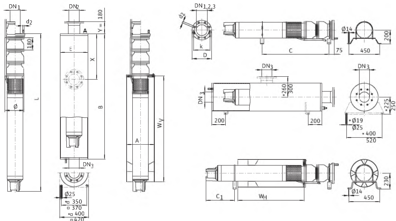
Чертёж с размерами Wilo-EMU K 126
