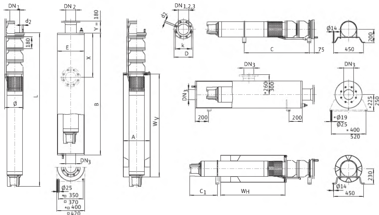
Чертёж с размерами Wilo-EMU K 127
