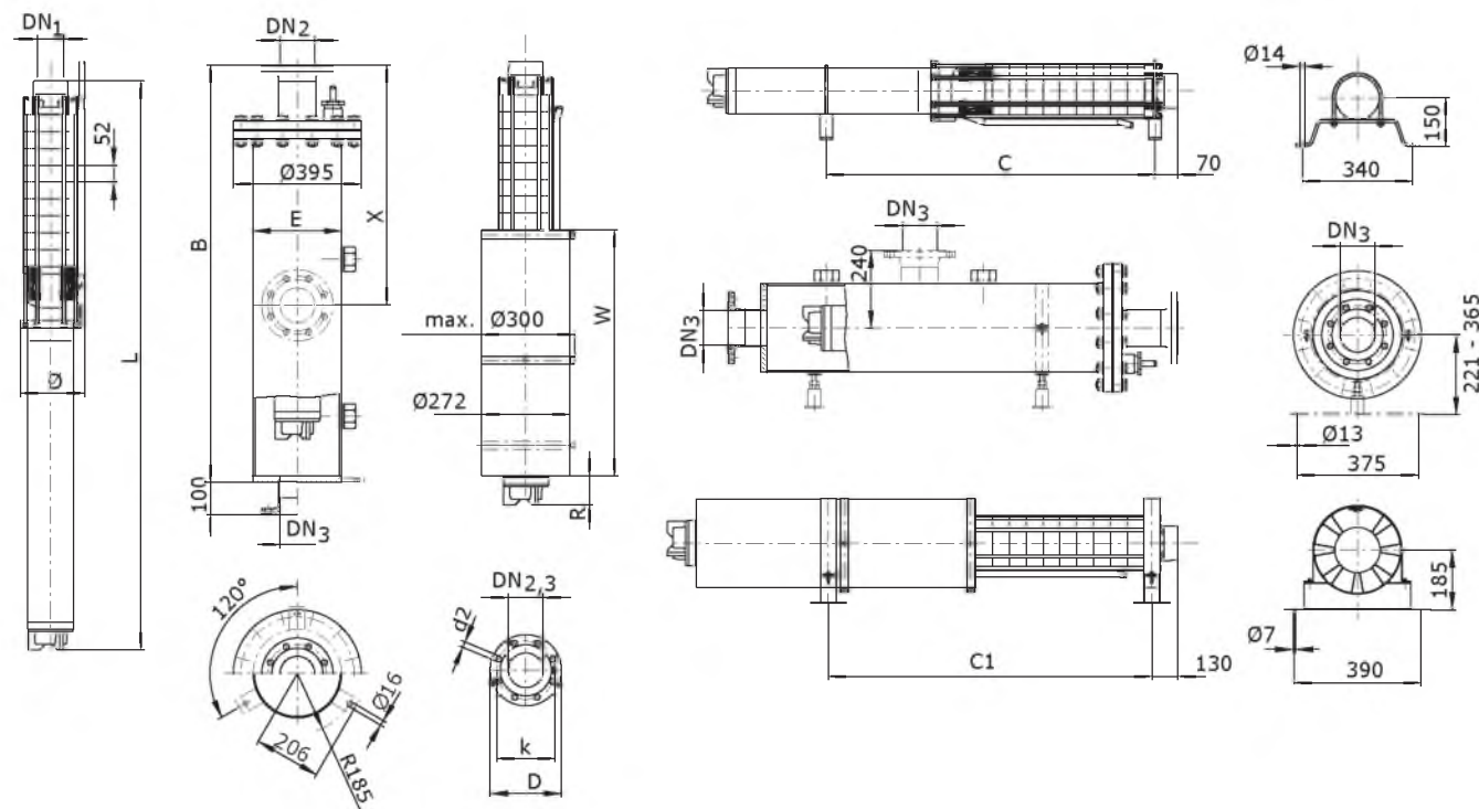
Чертеж с размерами Wilo-EMU NK 80
