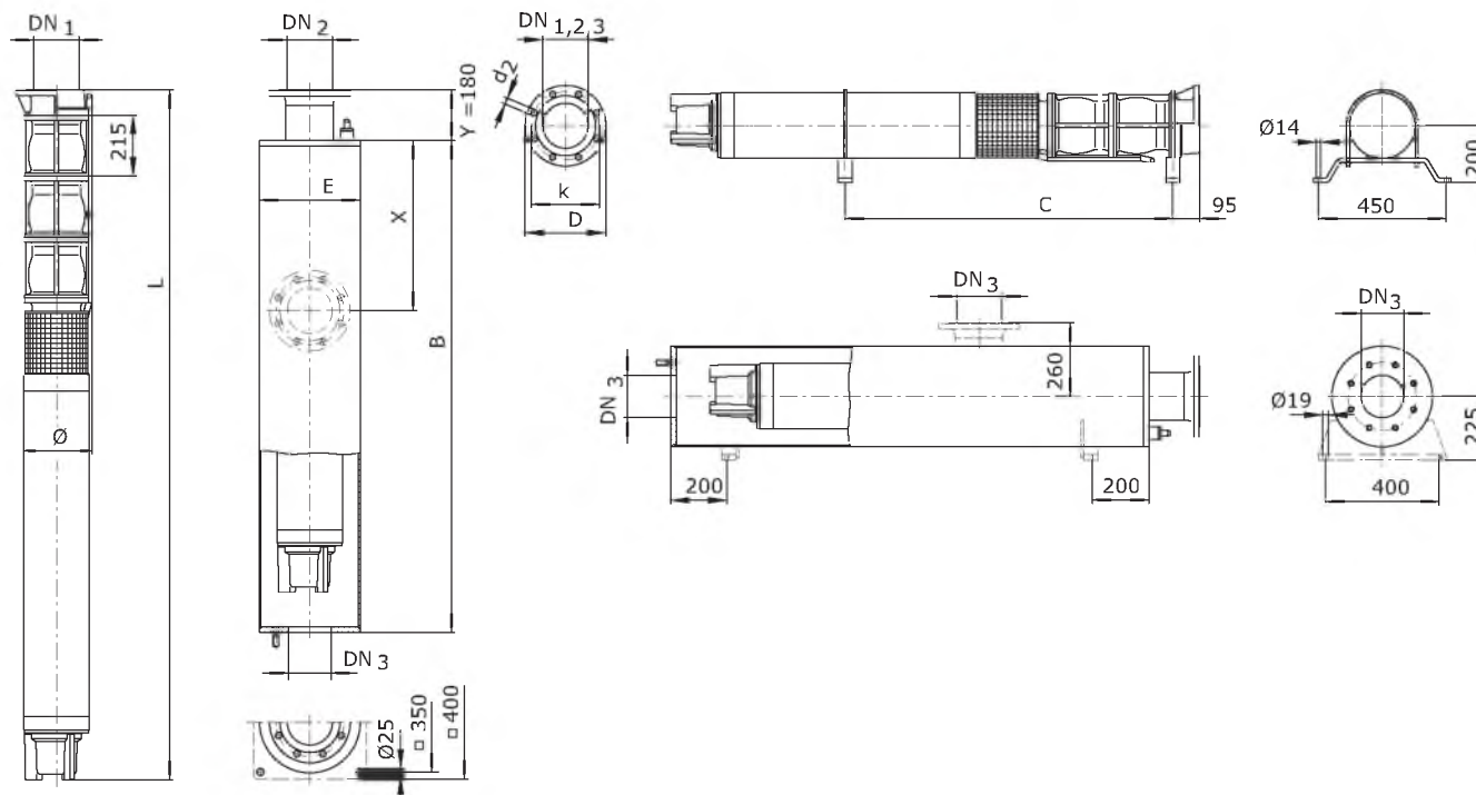
Чертеж с размерами Wilo-EMU SCH 200
