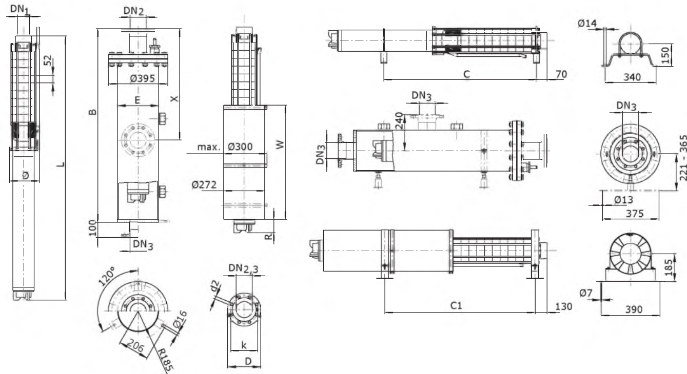
Чертеж с размерами Wilo-EMU NK 81
