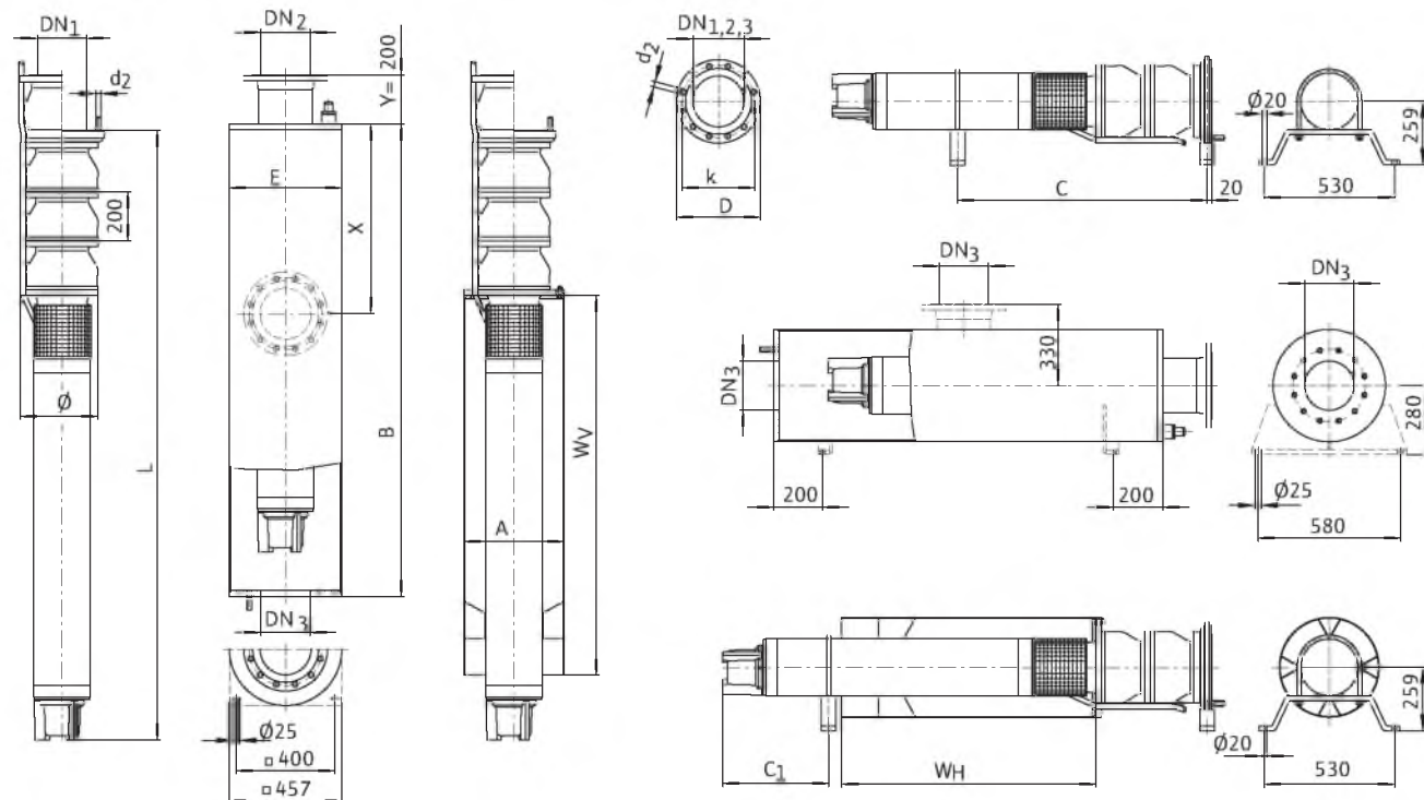
Чертёж с размерами Wilo-EMU K 146
