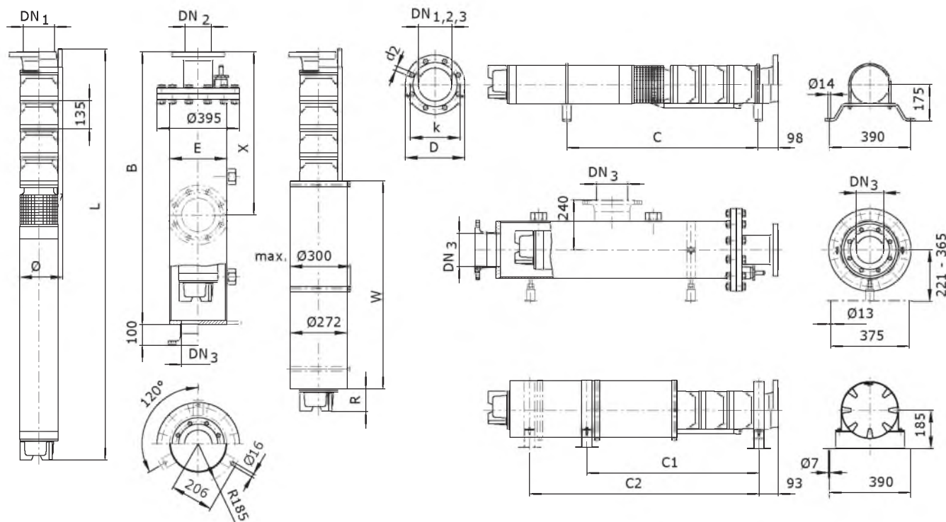
Чертеж с размерами Wilo-EMU NK 86
