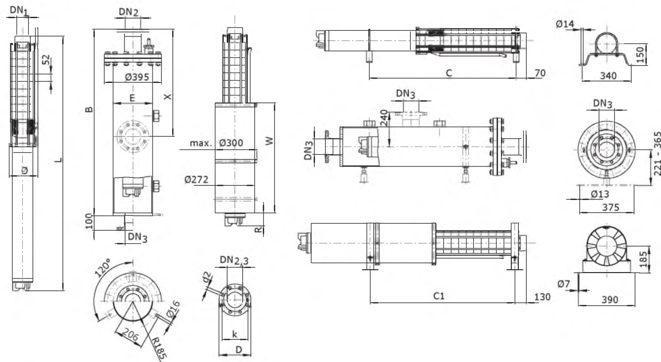
Чертёж с размерами Wilo-EMU NK 80
